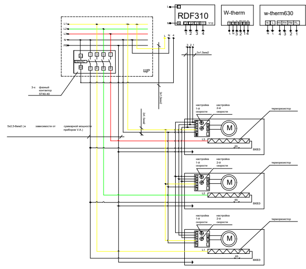
Схема подключения группы конвекторов ВКВЭ через контактор ST40-40 для 3-х фазной цепи 380В.
